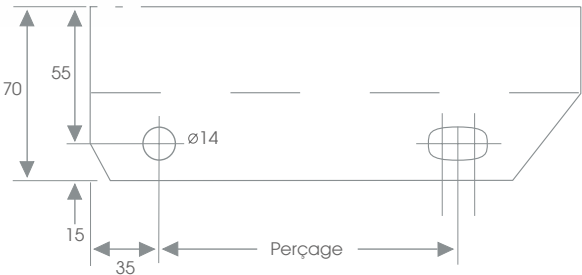
GABARIT DE PERÇAGE
