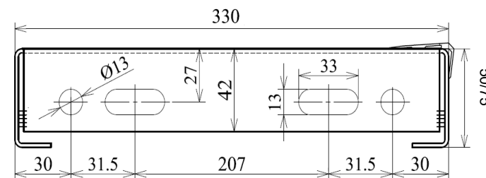
Perçage des goussets
