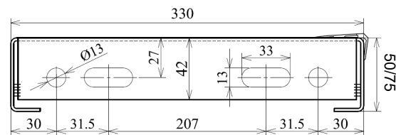
Perçage des goussets
