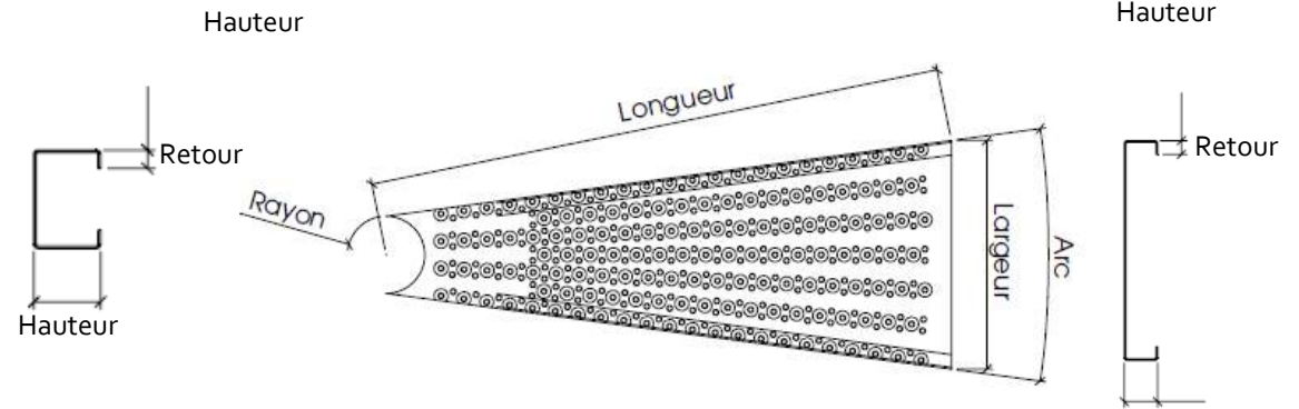
Exemple de marche balancée en triangle
