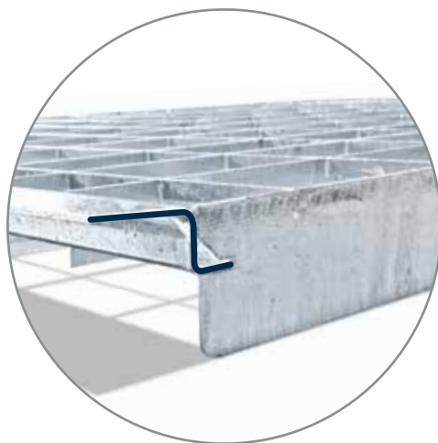
Le profil Z permet l'insertion du rayonnage.
